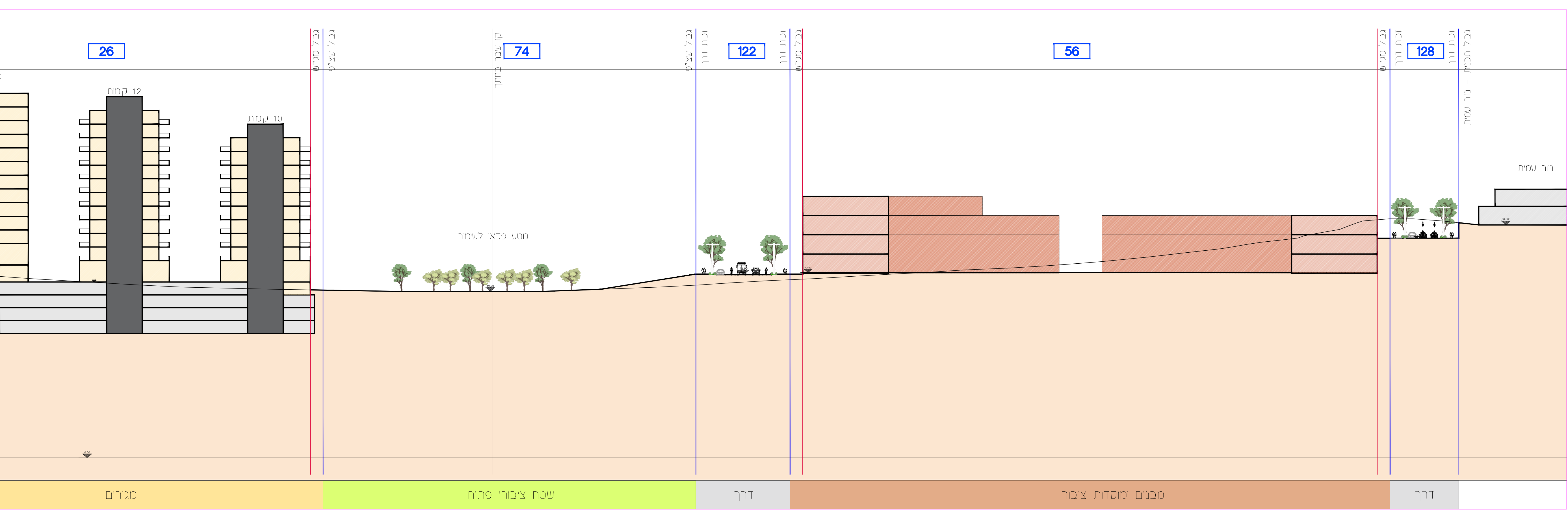
חתך ז-ז
